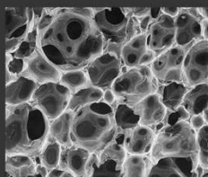
試料：ポリウレタン 加速電圧：10 kV 撮影倍率：×100
