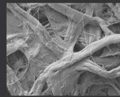
試料：紙表面 加速電圧：15 kV 撮影倍率：×500
