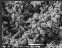
試料：酸化亜鉛 加速電圧：10 kV 撮影倍率：×10,000
