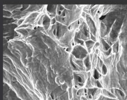
試料：アルミ疲労波面観察 加速電圧：15 kV 撮影倍率：×3,000
